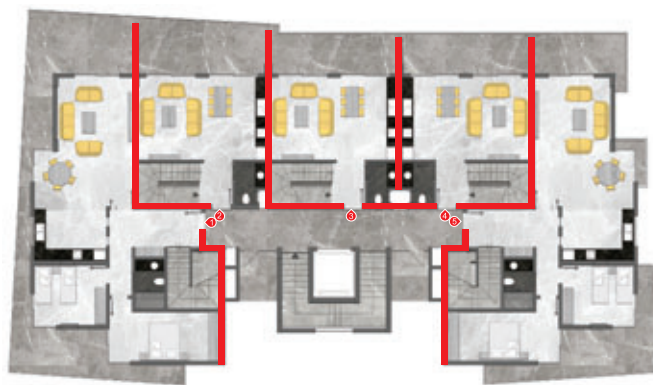
A BLOK DUBLEKS KAT PLANI
